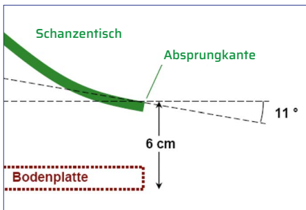
Skizze - Ausschnitt Schanzentisch
